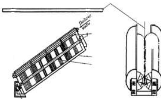
Рисунок 1.2 – Устройство моечной машины K7-ФМГ для туш свиней в шкуре после обескровливания и при мокром туалете
